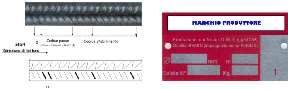
Figura 1: Esempio di marchio di laminazione e di etichetta.
