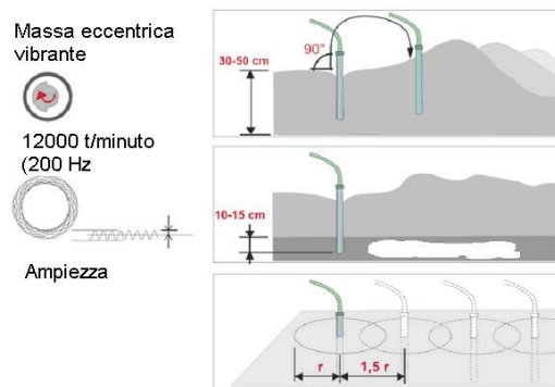
Figura 13: Caratteristiche dei vibratori interni.
