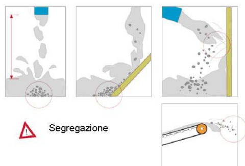
Figura 7: Errori nella posa in opera del calcestruzzo.
