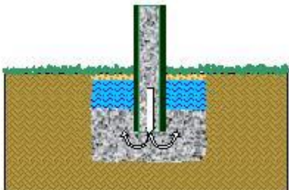
Figura 10: Getto di calcestruzzo in presenza di acqua.
